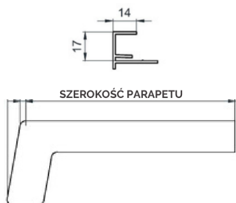
PRZEKRÓJ ZAŚLEPKI
