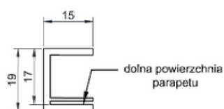
PRZEKRÓJ ZASŁEPKI
