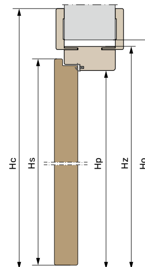
Panel pojedynczy
