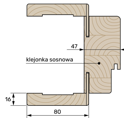
Panel pojedynczy
