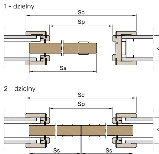
System wewnętrzścienny
